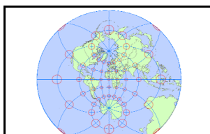
Stereographic 平射図法
