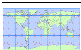
Patterson パターンソン図法
