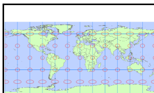
Plate Carree 正方形図法
