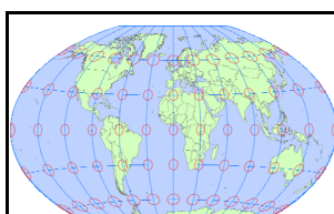
Winkel Tripel ヴィンケル図法 (第3図法)
