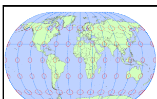
Winkel II ヴィンケル図法 (第2図法)
