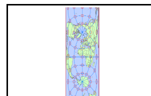
Transverse Cylindrical Equal Area 横正横円筒図法
