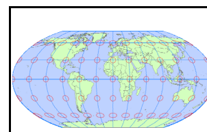
Wagner V ワグナー図法 (第5図法)
