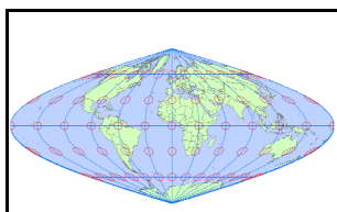
Sinusoidal サンソン図法 (正弦曲線図法)
